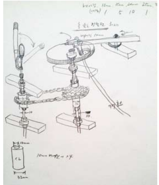
«Cancellation Machine»(Drawing)
